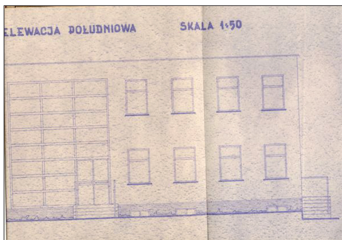
Elewacja południowa projektowanego budynku biurowo - warsztatowego ADM 4 w Giżycku, 1970 r. z archiwum MBP w Giżycku
